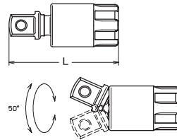
2771 Universal Joint Articulación Universal
