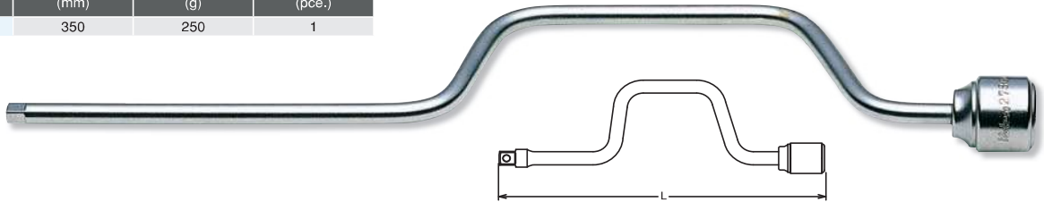
2780 Speed Handle Manivela Rápida
